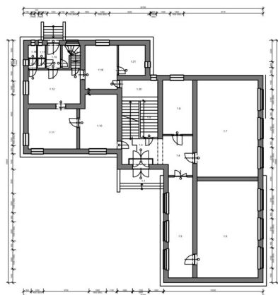
Pôdorys 1 NP
