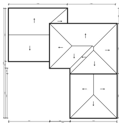
Pôdorys striech
