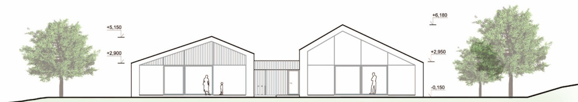
ZÁPADNÝ POHLAD
